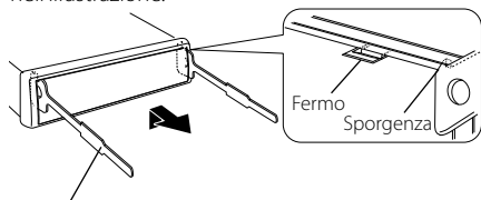
Accessorio② Attrezzo per la rimozione
